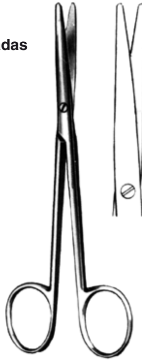
LEXER 12-2220 16 cm, 6¼"
